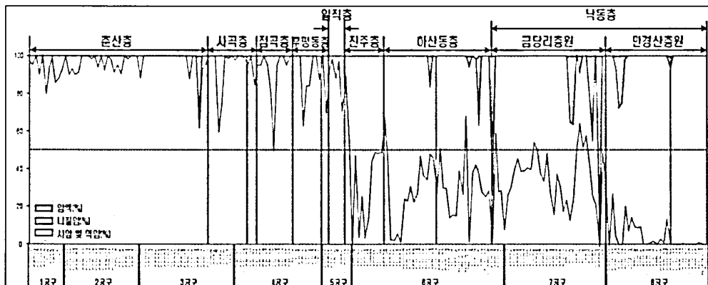
&lt; 영천~상주간 고속도로 분포 총균 지질종단도 &gt;
