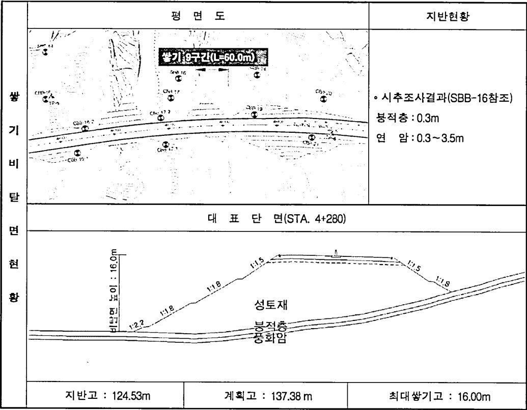
(10) 쌓기 9구간 (STA. 4+250~4+310, L=60.0m)
