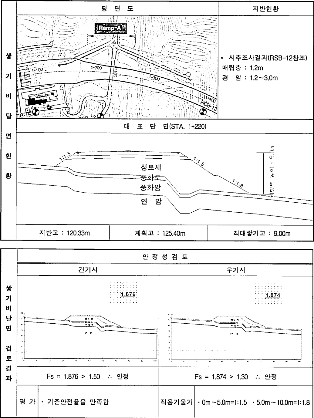
(21) Ramp - A (STA. 1+190 ~ 1+270, L=80.0m)
