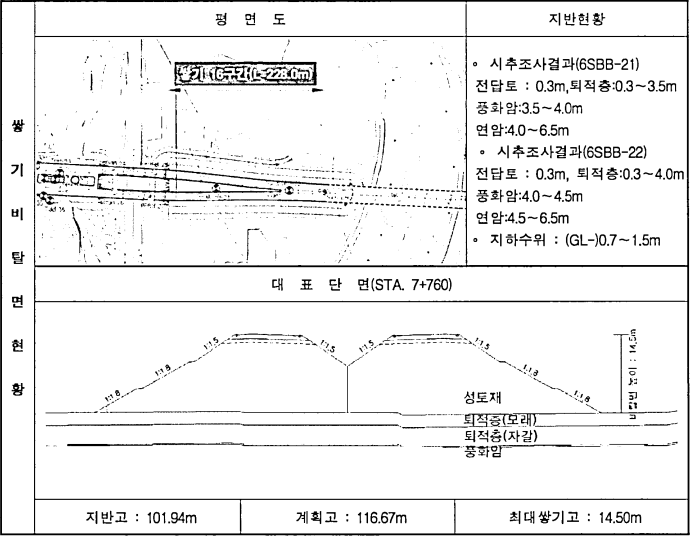
(17) 쌓기 16구간 (STA. 7+750~7+980, L=228m)
