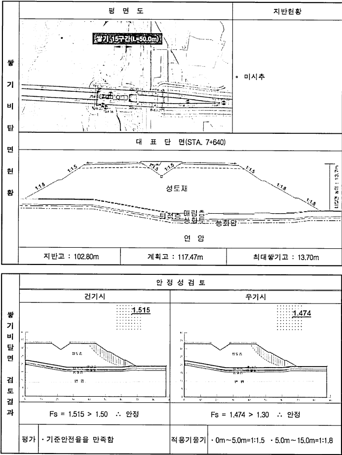
(16) 쌓기 15구간 (STA. 7+610~7+660, L=50m)
