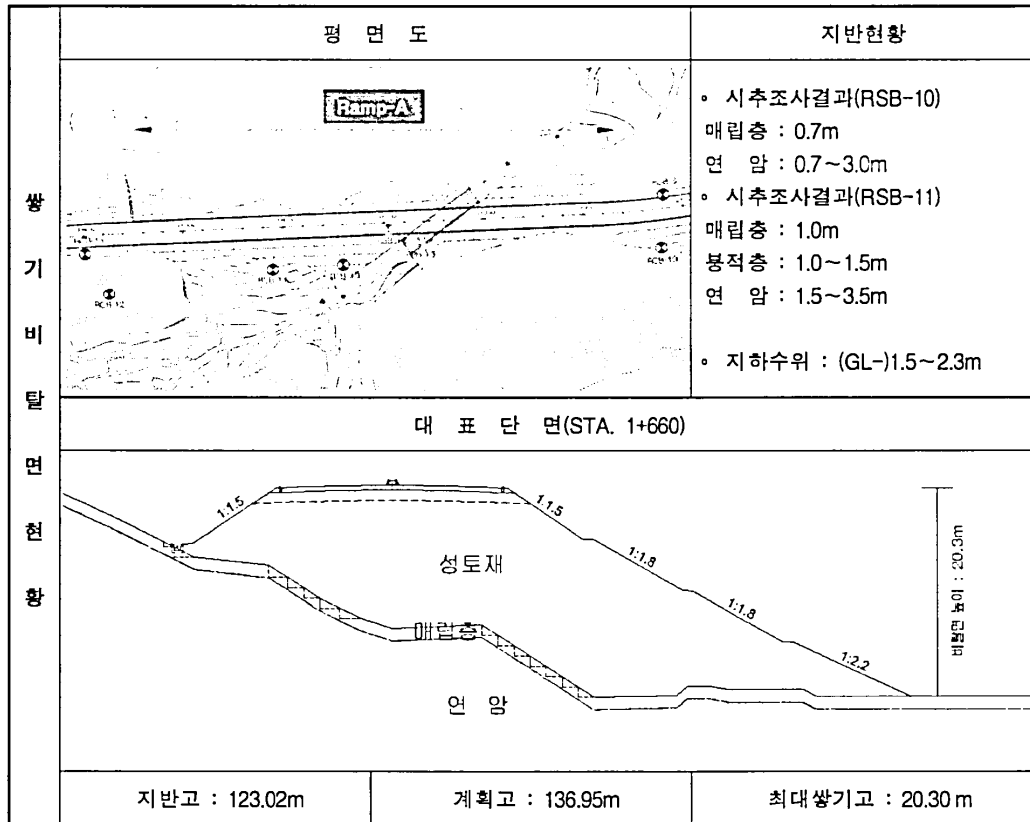
(22) Ramp - A (STA. 1+450 ~ 1+930, L=480.0m)
