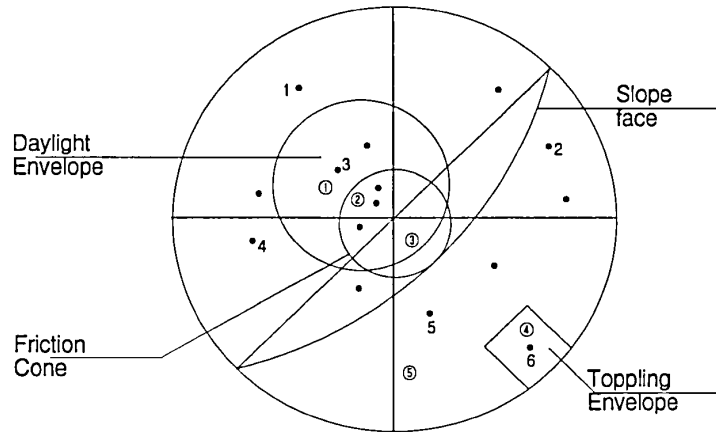
< 평사투영에 의한 암반비탈면의 안정성 평가 >
