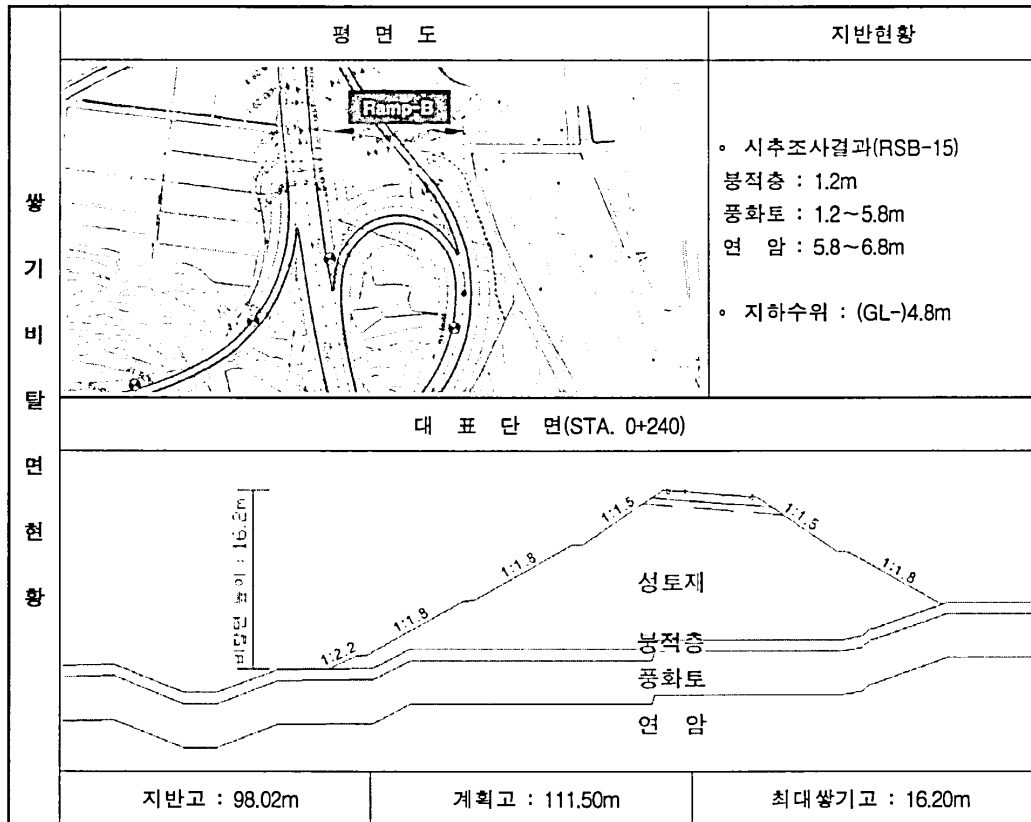
(24) Ramp - B (STA. 0+160~0+367.7, L=207.7m)
