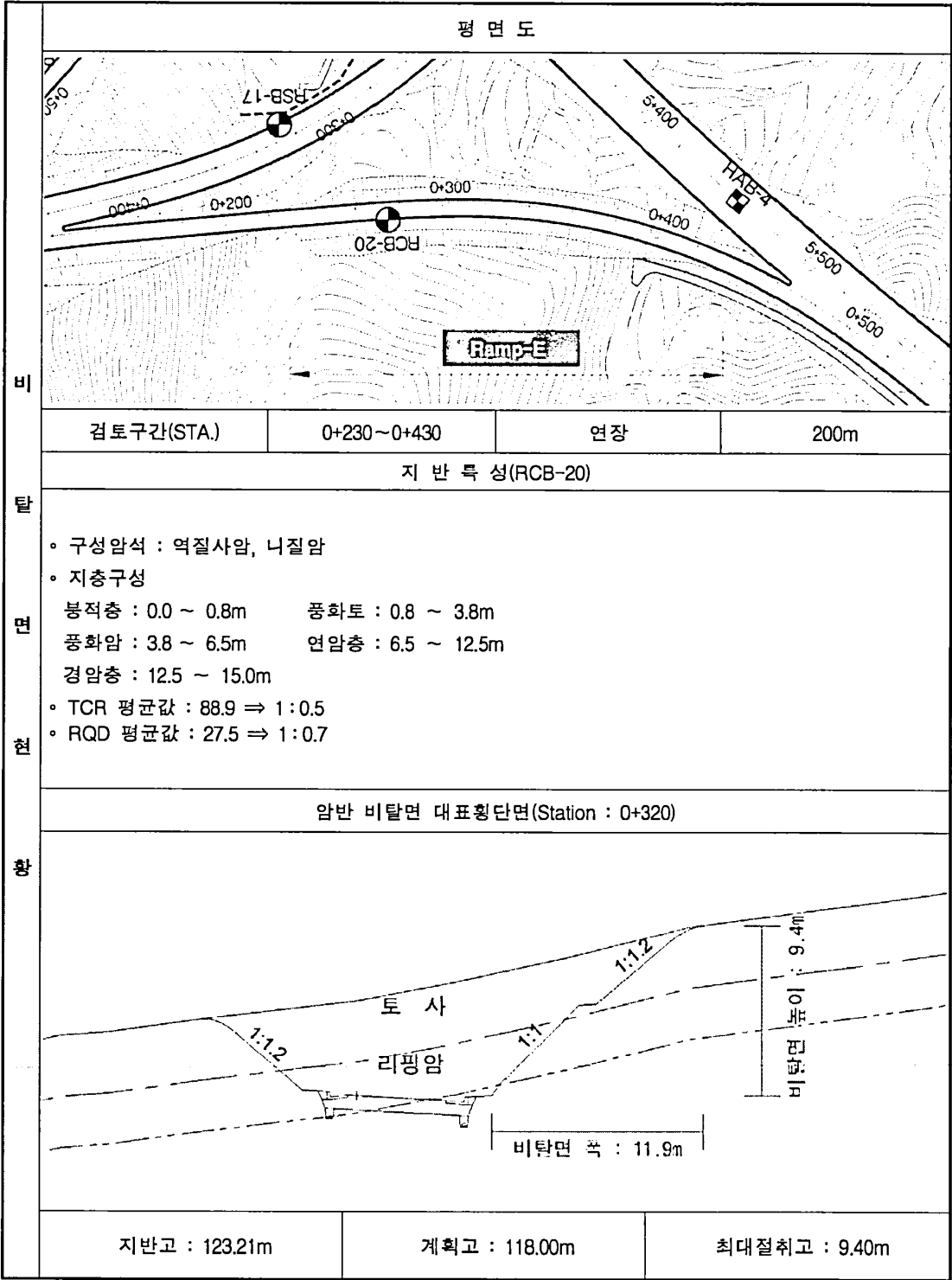
(23) Ramp -E (STA. 0+230~0+430)
