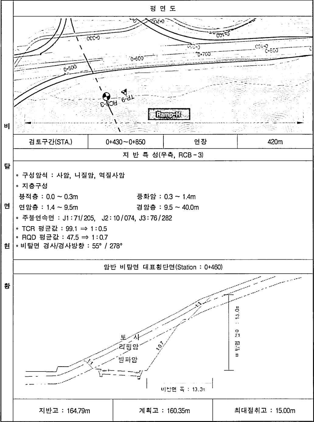
(26) Ramp-H(STA. 0+430~0+850)
