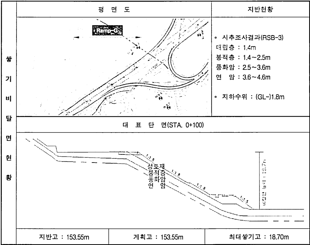
(28) Ramp-G (STA. 0+020~0+290, L=270.0m)
