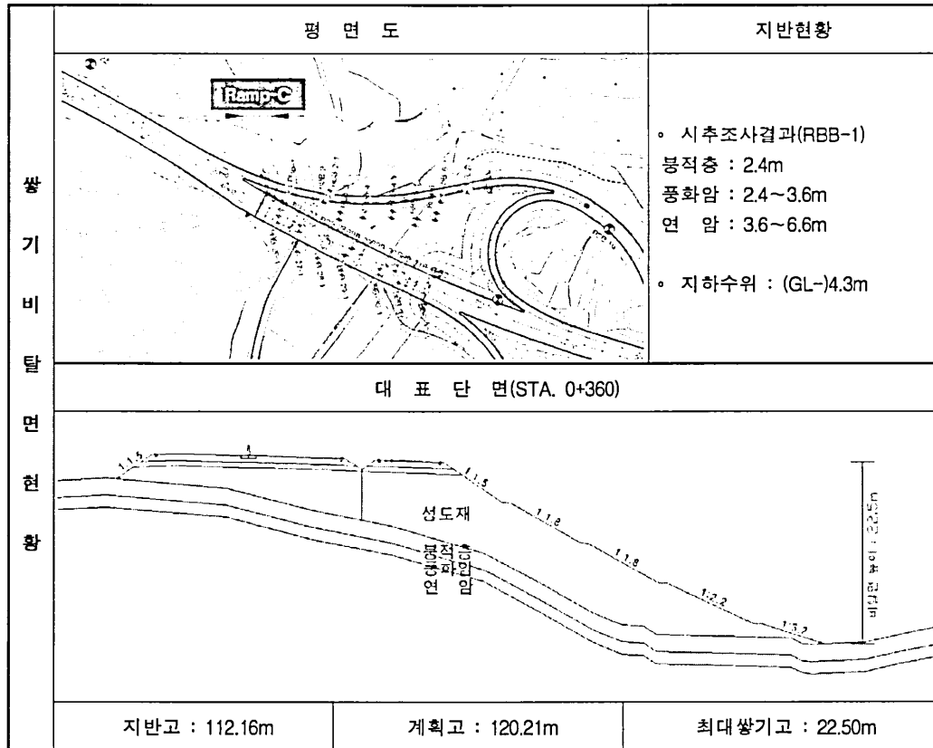
(26) Ramp - C (STA. 0+353~0+380, L=27.0m)
