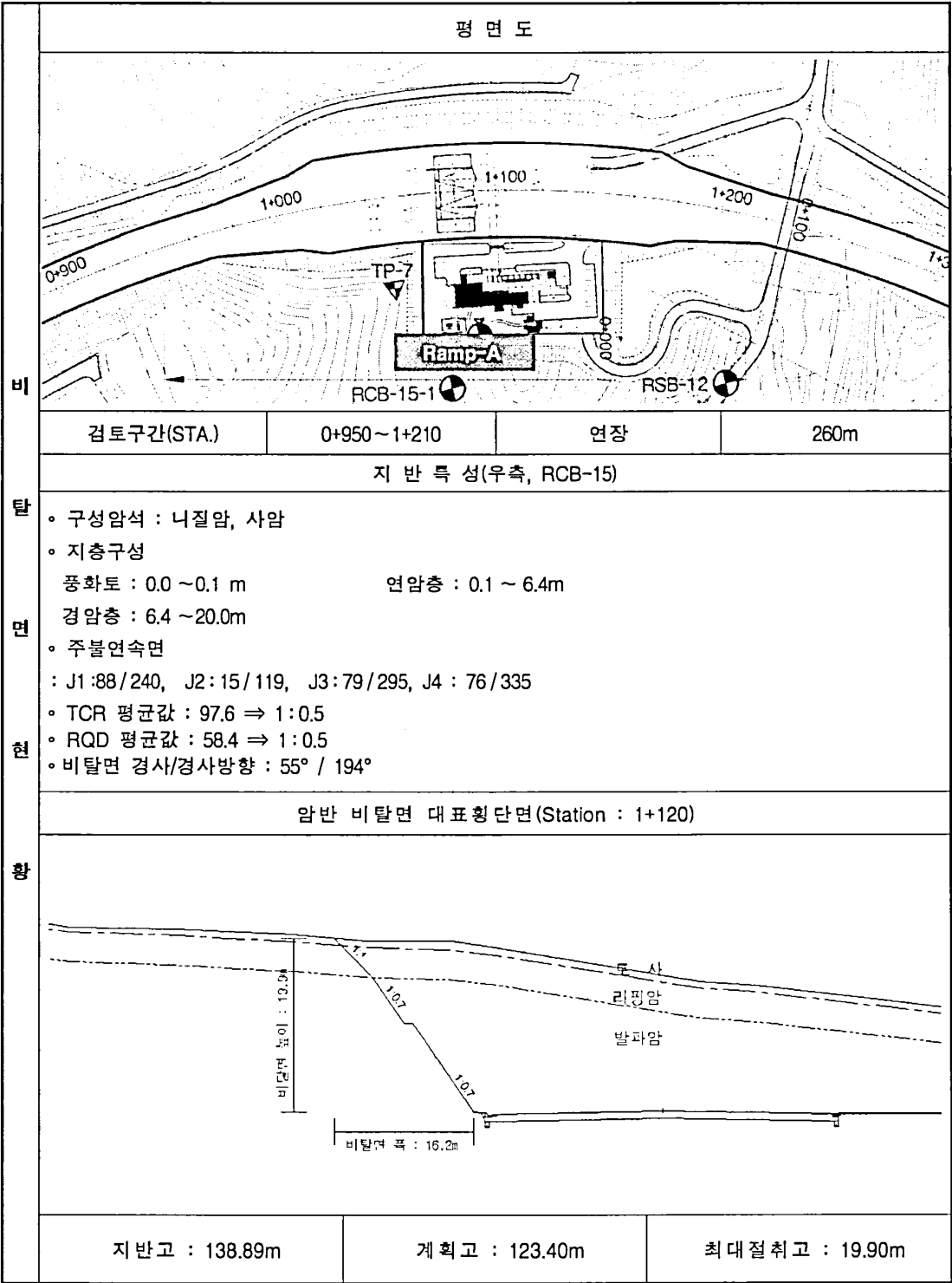
(17) Ramp - A(STA. 0+950~1+210)
