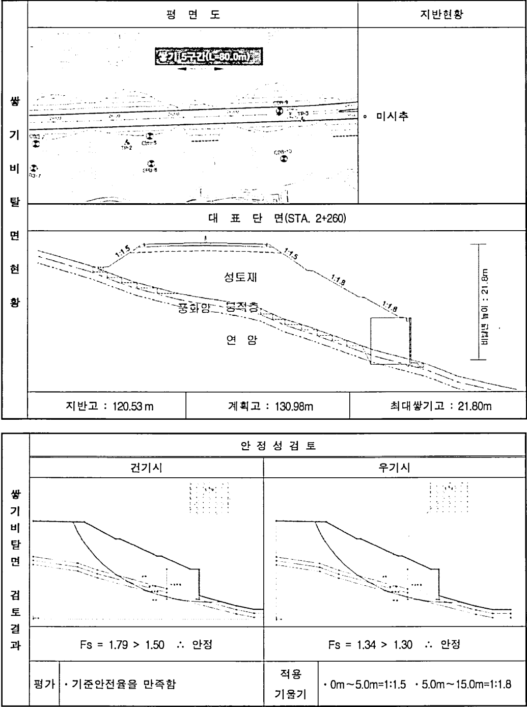
(5) 쌓기 5구간 (STA. 2+210~2+290, L=80.0m)
