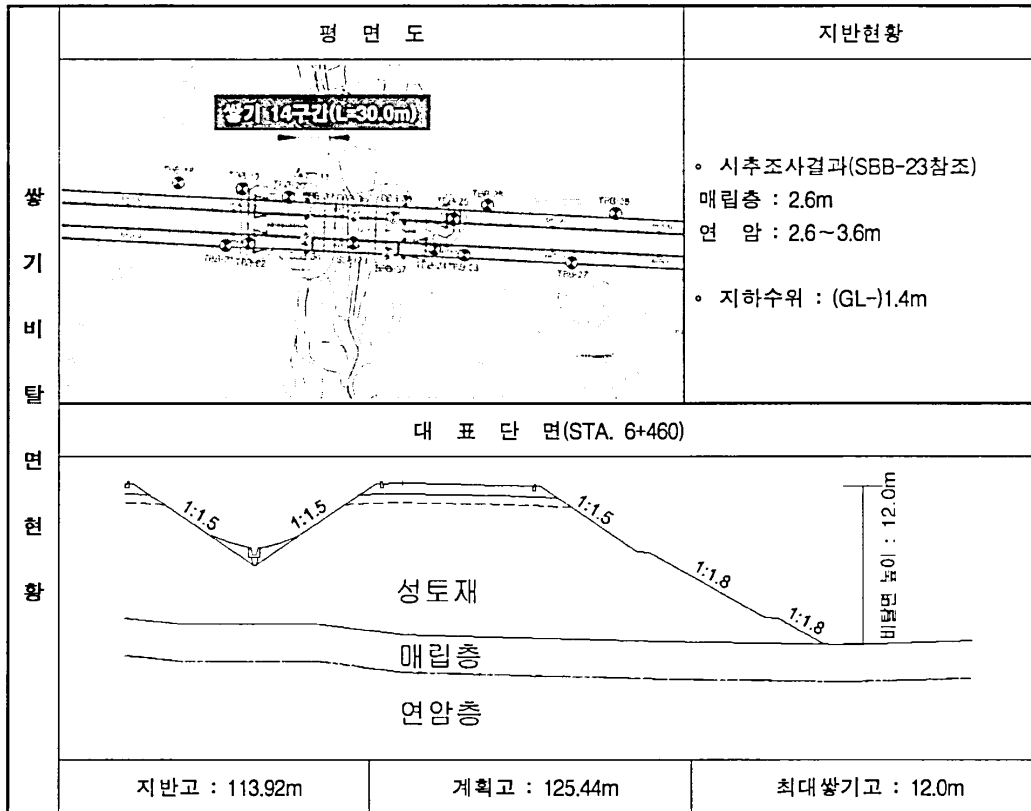
(15) 쌓기 14구간 (STA. 6+440~6+470, L=30.0m)
