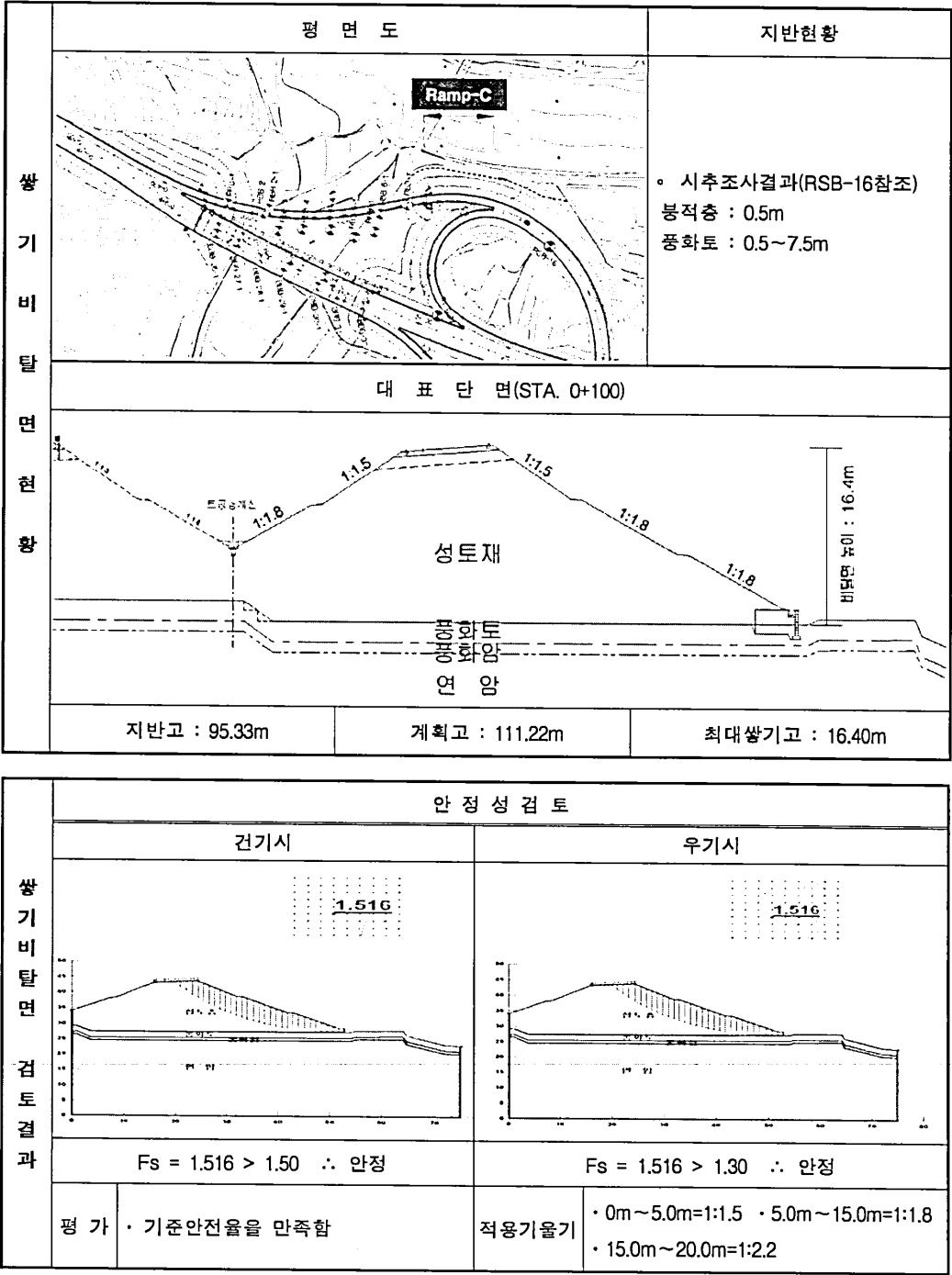
(25) Ramp - C (STA. 0+040~0+113, L=73m)
