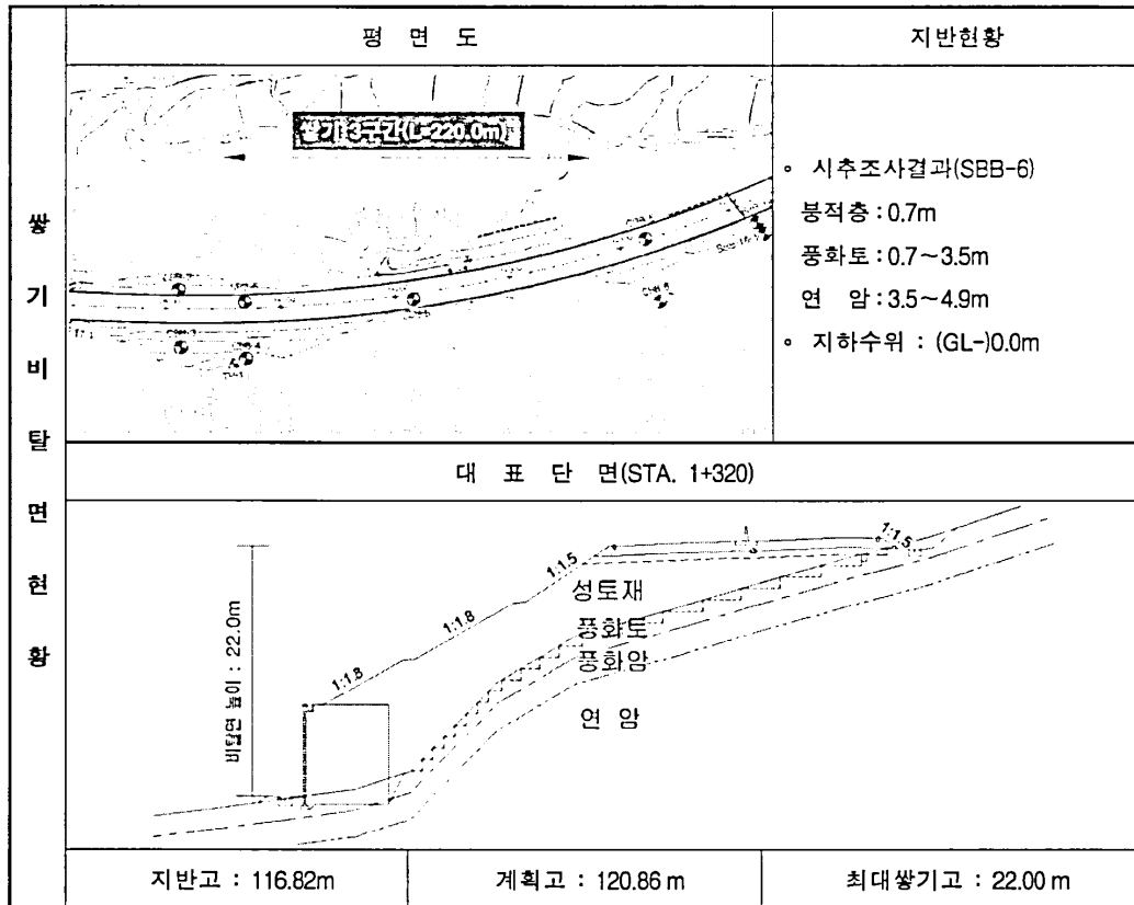
(3) 쌓기 3구간 (STA. 1+150~1+370, L=220.0m)
