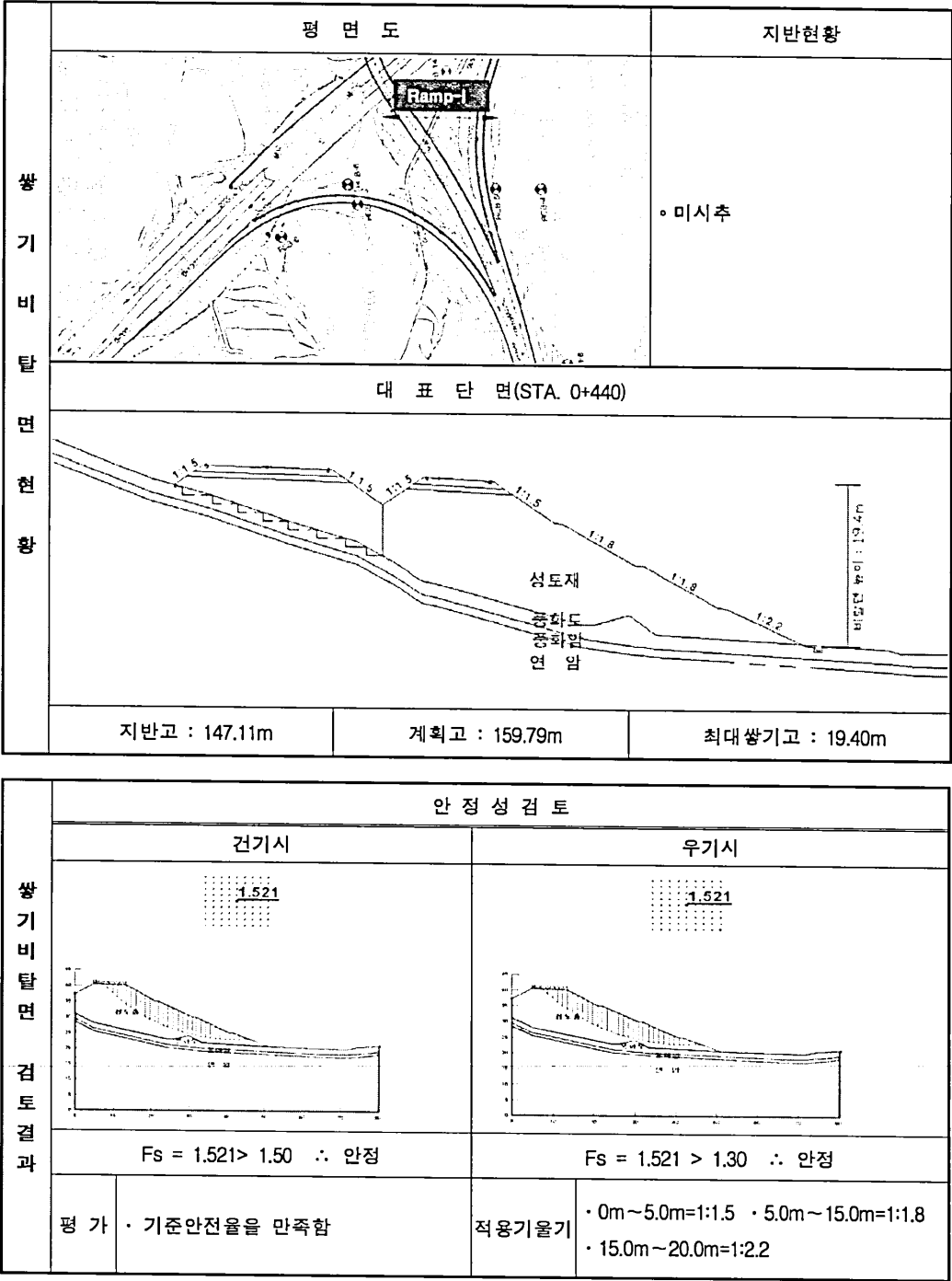
(31) Ramp - I (STA. 0+330~0+500, L=170.0m)
