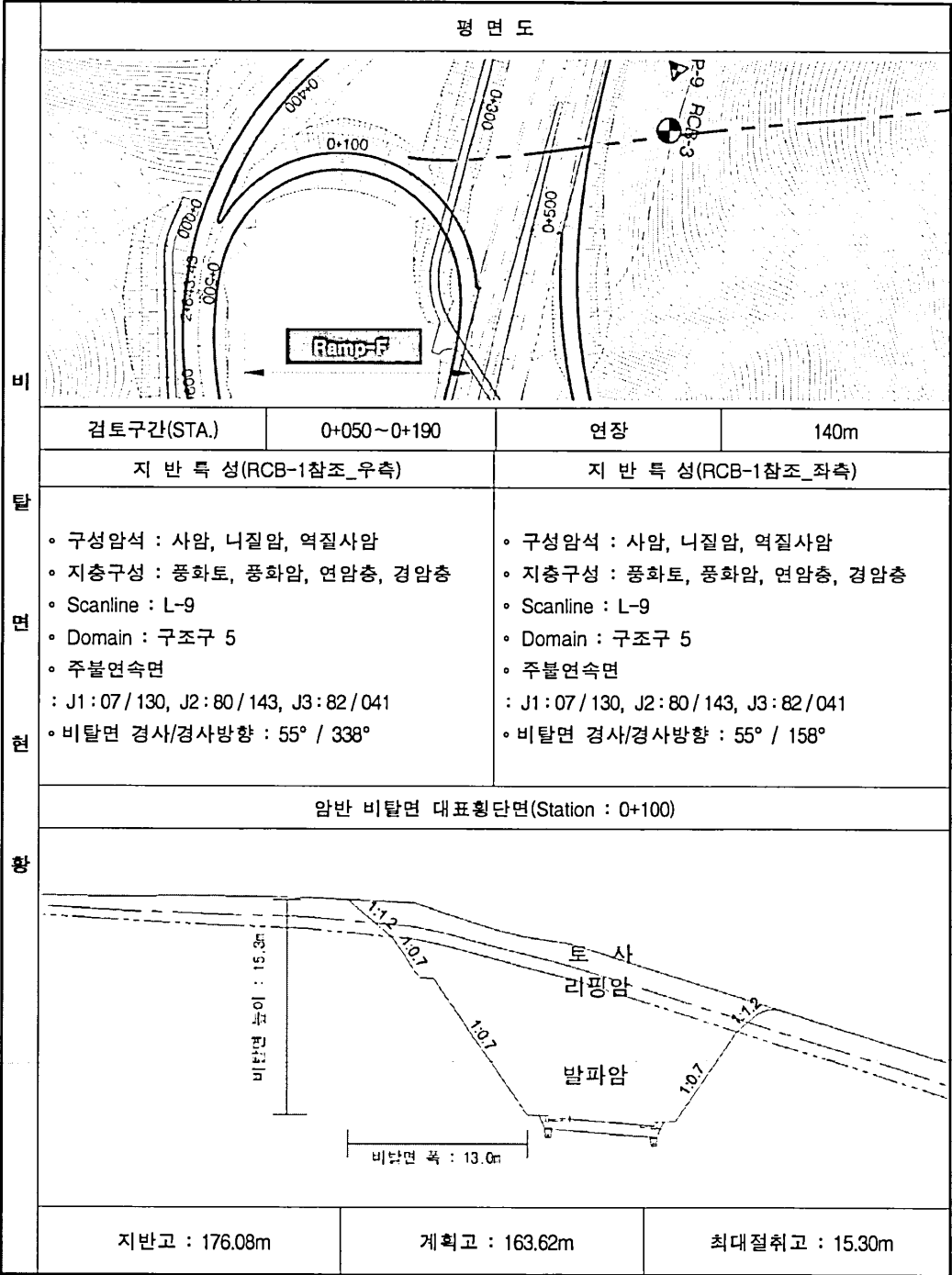
(24) Ramp -F (STA. 0+050~0+190)
