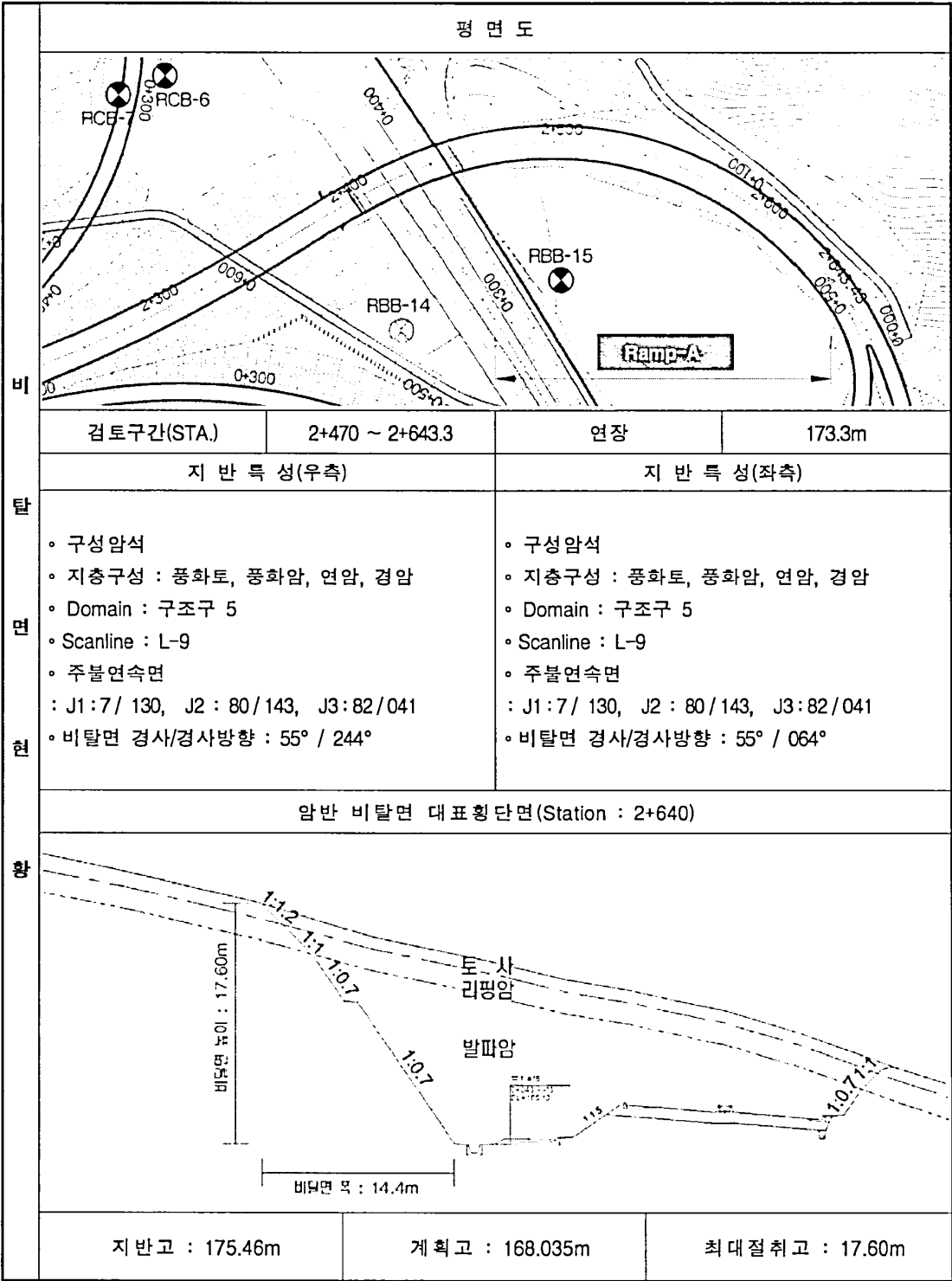
(21) Ramp - A(STA. 2+470 ~ 2+643.3)
