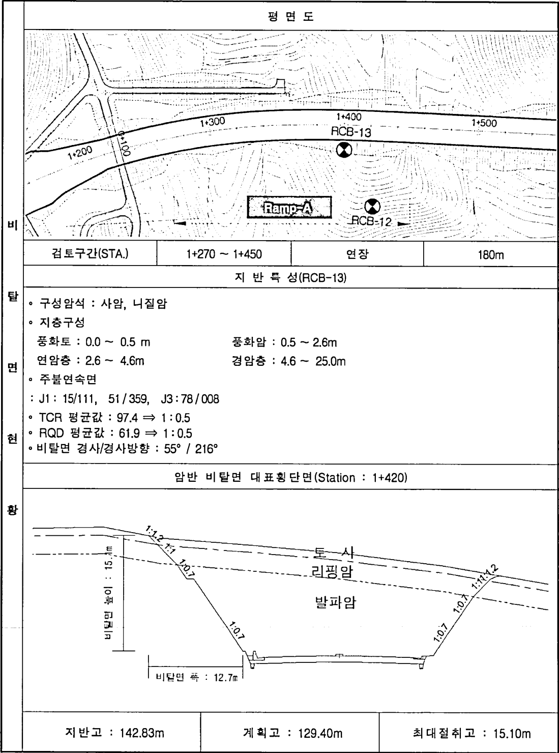
(18) Ramp - A(STA. 1+270 ~ 1+450)
