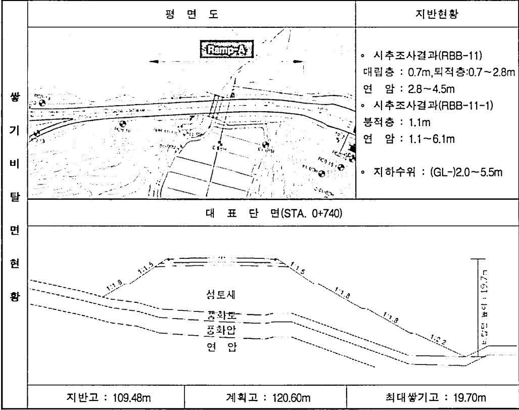
(20) Ramp - A (STA. 0+680~0+970, L=290m)
