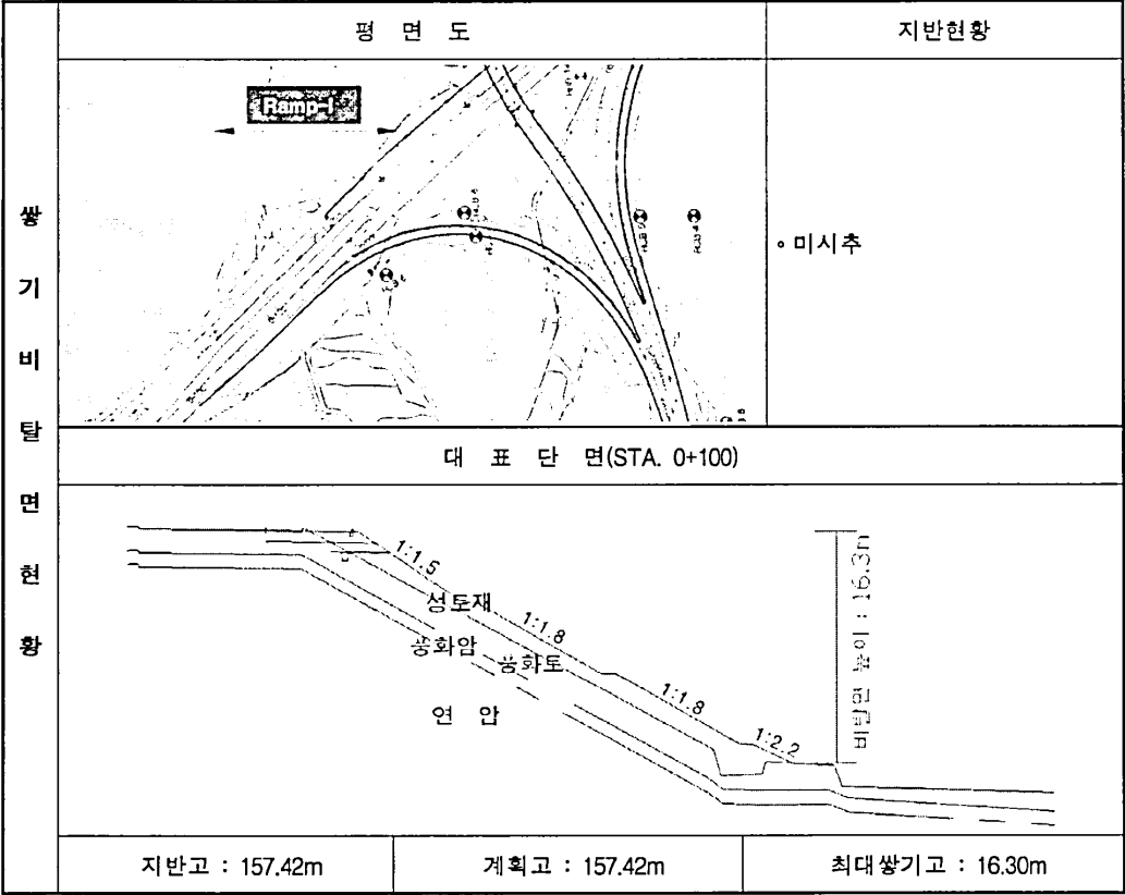
(30) Ramp - I (STA. 0+020~0+230, L=210.0m)
