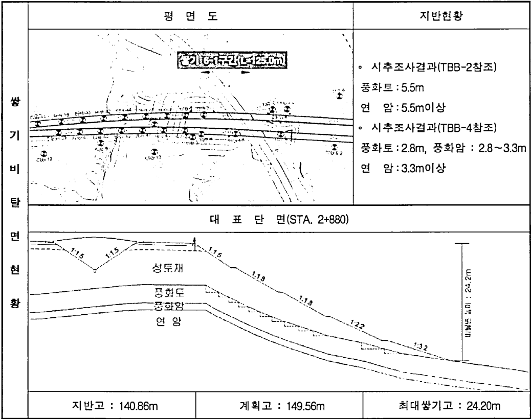
(7) 쌓기 6-1구간 (STA. 2+825~2+950, L=125.0m)
