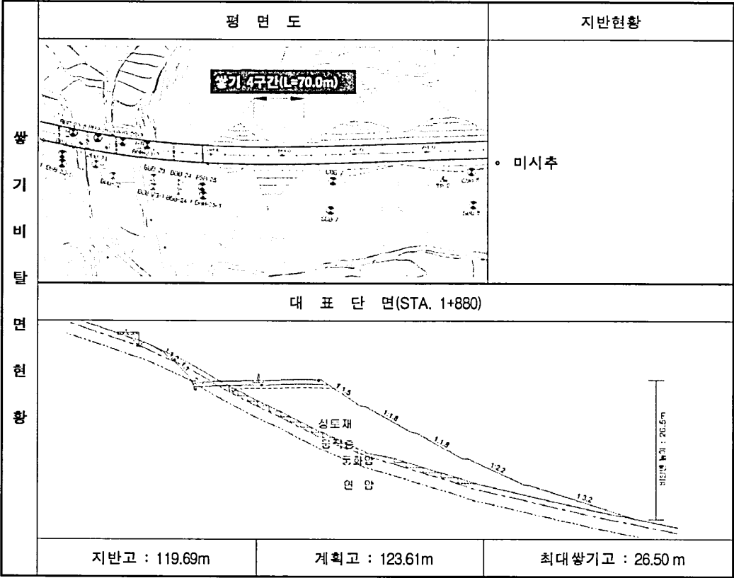
(4) 쌓기 4구간 (STA. 1+860~1+930, L=70.0m)
