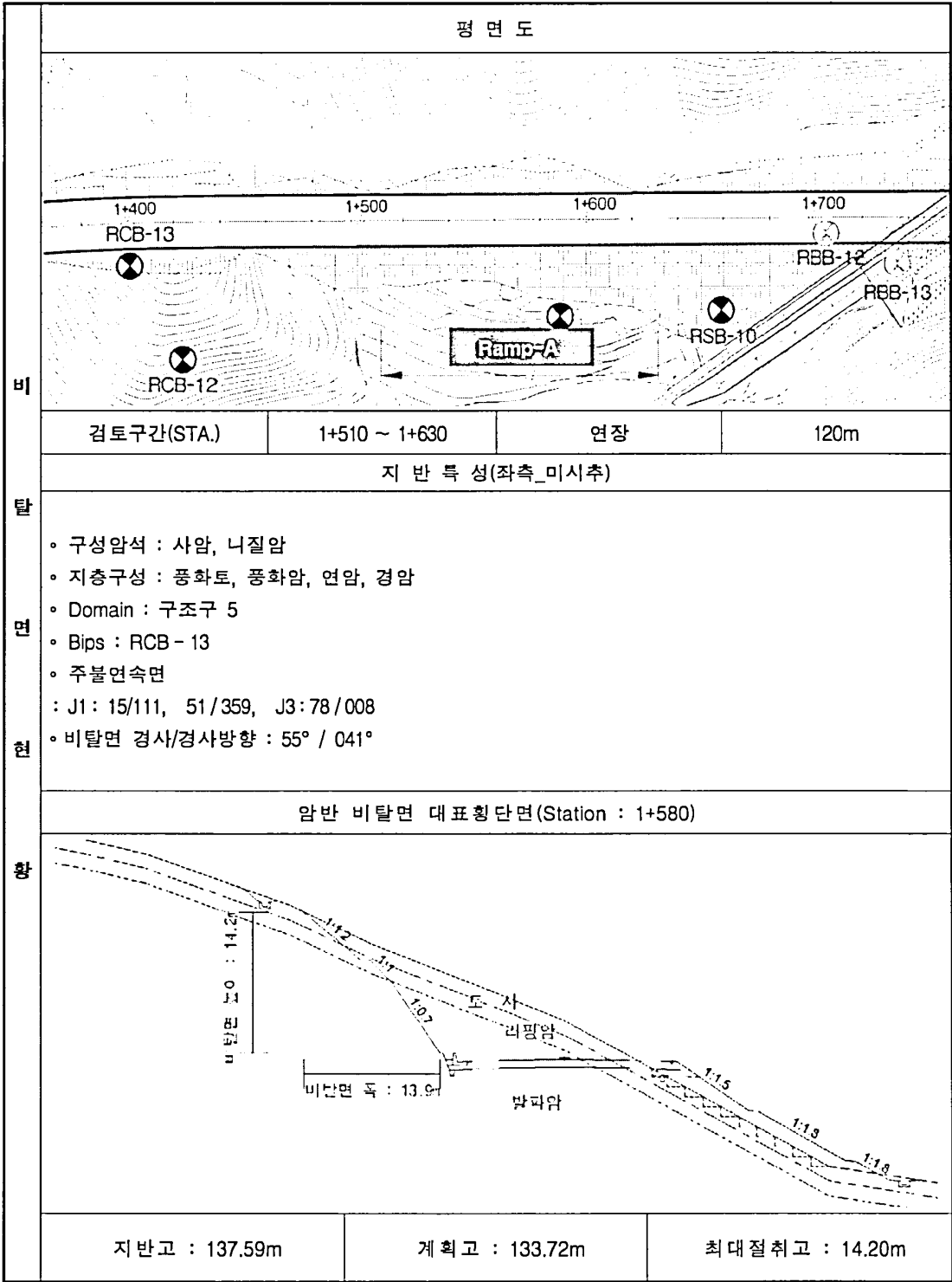
(19) Ramp - A(STA. 1+510 ~ 1+630)
