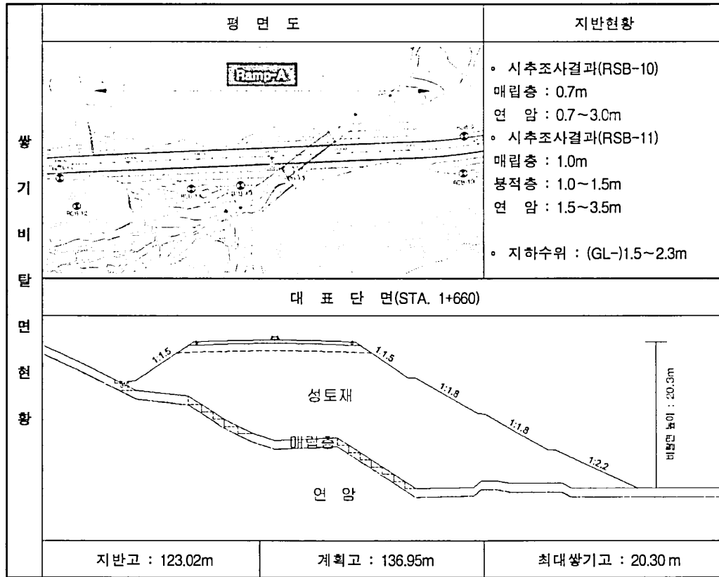
(22) Ramp - A (STA. 1+450 ~ 1+930, L=480.0m)
