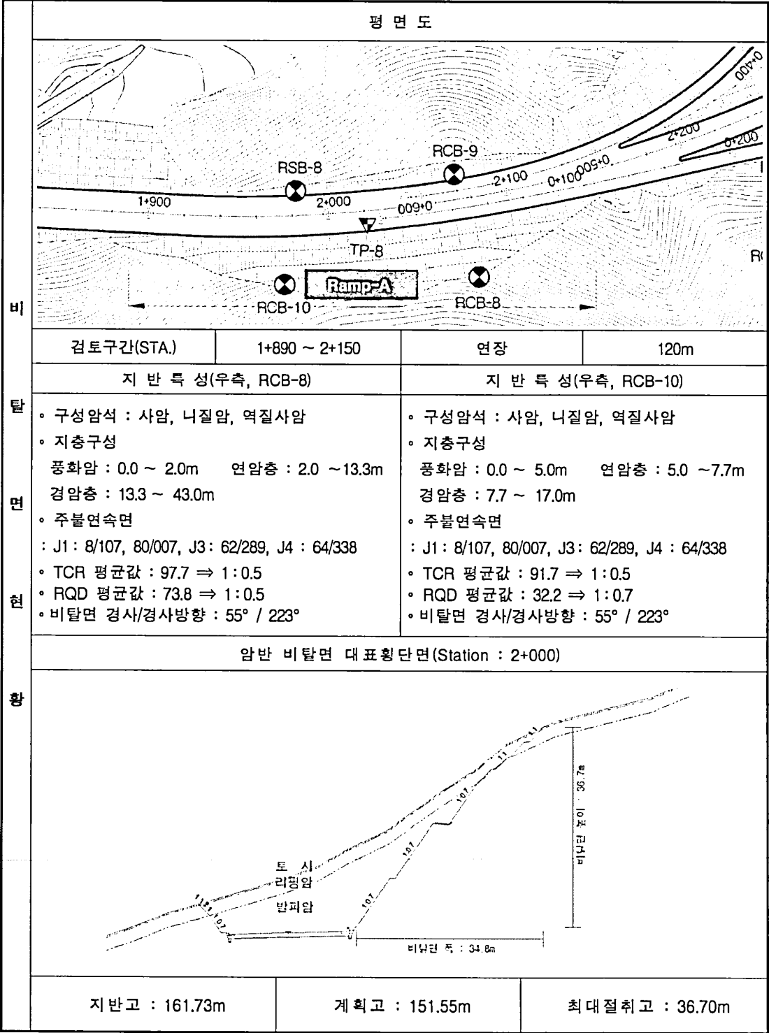
(20) Ramp - A(STA. 1+890 ~2+150)
