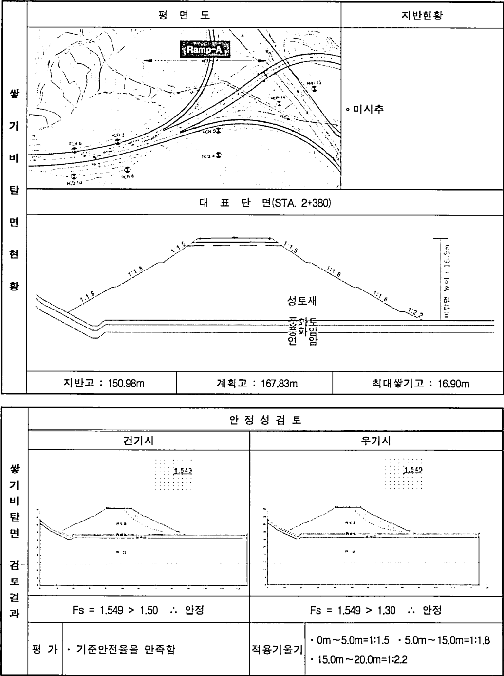
(23) Ramp - A (STA. 2+130~2+401, L=271.0m)
