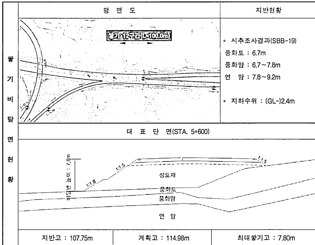
(13) 쌓기 12구간 (STA. 5+550~5+650, L=100.0m)
