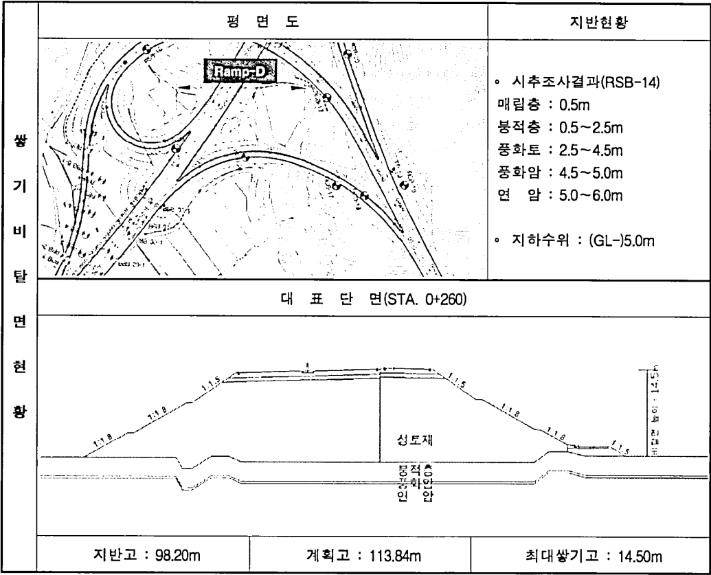
(27) Ramp - D (STA. 0+260~0+450, L=190.0m)
